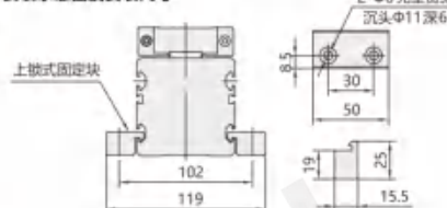
安装示意图及安装尺寸
