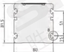
A-A View(2:1)
